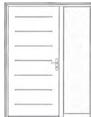
ÉQUATION LARGEUR MAXIMUM AVEC FIXE H 2150 L 1600 FERRAGE UNIQUEMENT SUR DORMANT
