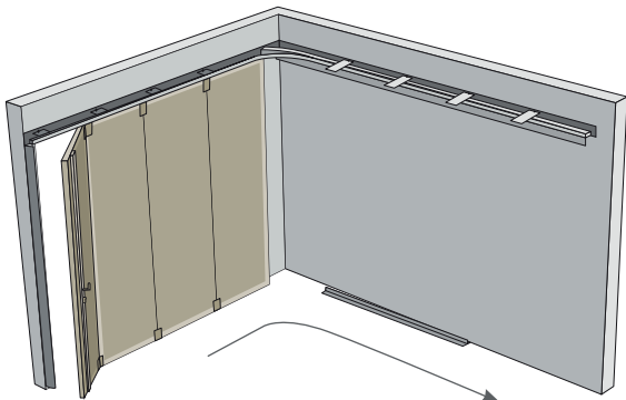
Portillon côté fermeture
