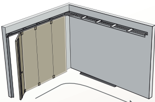
Vue intérieure avec portillon côté fermeture
