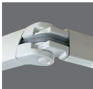
Bras à double câbles gainés Testés à 20 000 cycles.
