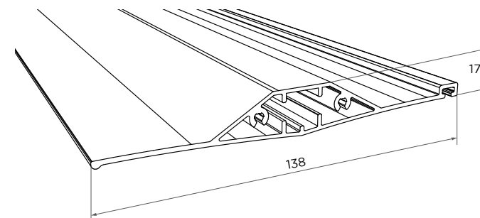
Coupe d'une lame - Dimensions en mm
