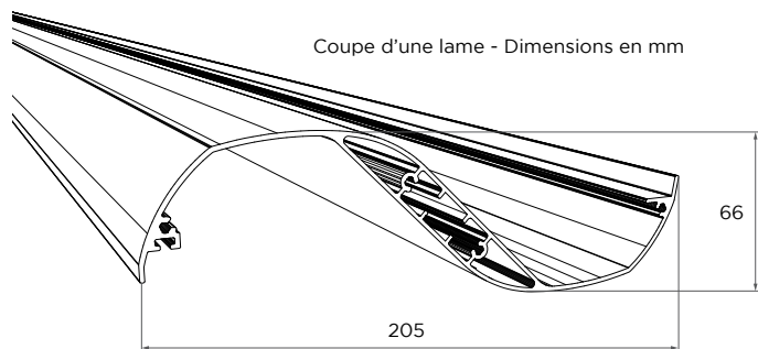
Lame ondulée en aluminium extrudé thermolaqué, de 205 x 66mm.
